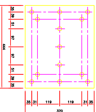
PIEZA 299 ESCALA 1:5 R. 370 x 10 x 444
