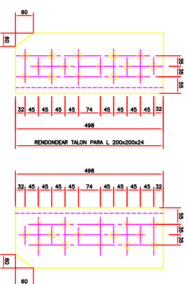
PIEZA 281 ESCALA 1:5 L 200 x 200 x 24 H Lq.=498
